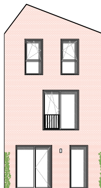
Achtergevel
